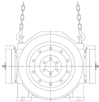
吊装示意图
