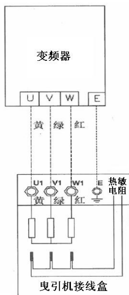
主回路接线图
